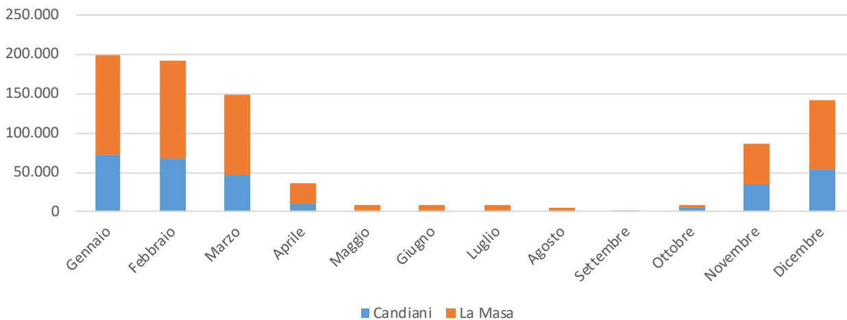
Figura 38. andamento mensile di consumo gas naturale [sm³], Sede Milano Bovisa
