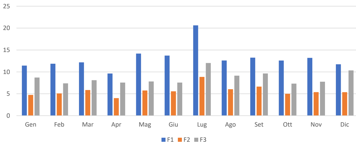
Consumo Energia Elettrica per Fascia - [MWh/mese]
