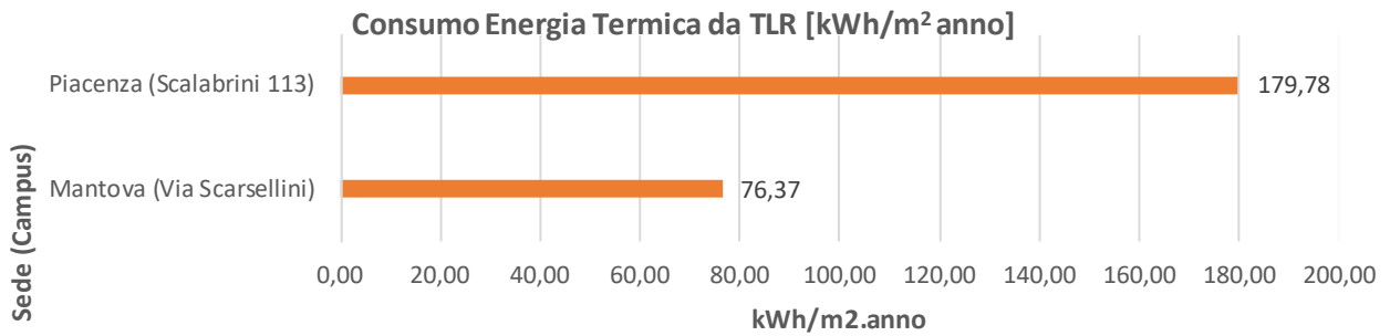
Figura 116. KPI consumo Energia Termica a livello di Campus
