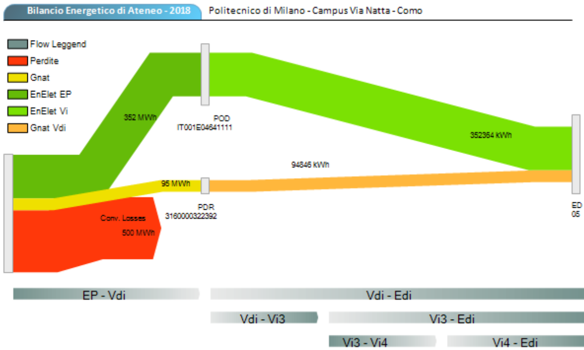
Figura 51. Diagramma di flusso dei vettori energetici, Campus via Natta
