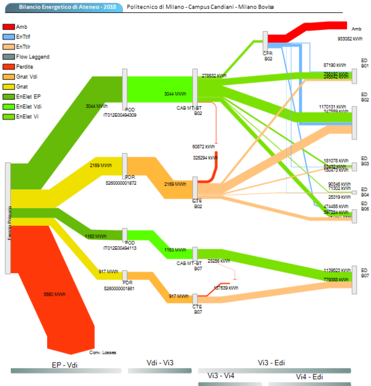
Figura 39. Diagramma di flusso dei vettori energetici, Campus Candiani
