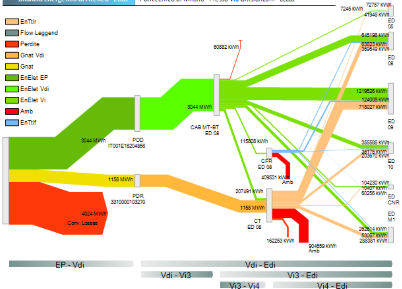
Figura 69. Diagramma di flusso dei vettori energetici, Campus Via Ghislanzoni
