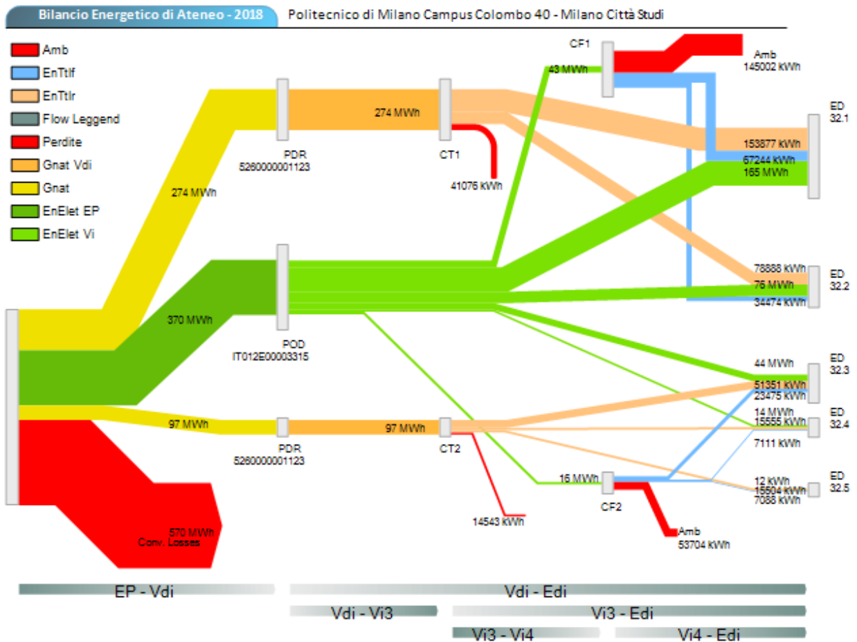
Figura 28. Diagramma di flusso dei vettori energetici, Plesso Leonardo 26 - Colombo 40
