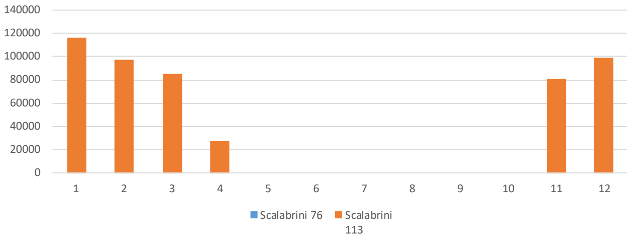
Figura 86. andamento mensile consumo Energia Termica da TLR [kWh], Sede Piacenza
