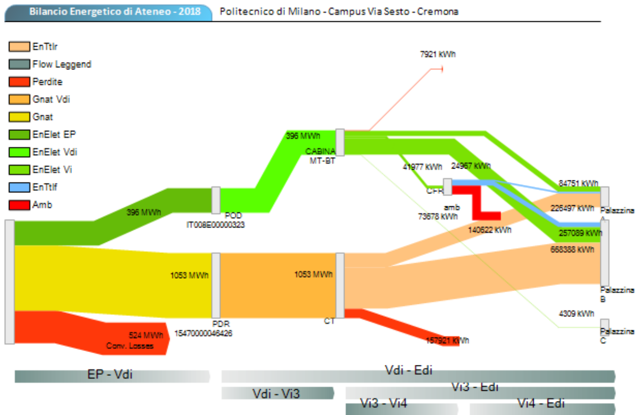
Figura 60. Diagramma di flusso dei vettori energetici, Campus via Sesto
