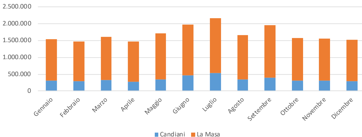
Figura 35. andamento mensile di consumo energia elettrica [MWh], Sede Milano Bovisa
