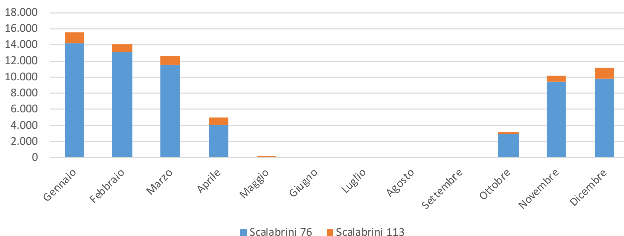
Figura 84. andamento mensile consumo gas naturale [Sm³], Sede Piacenza
