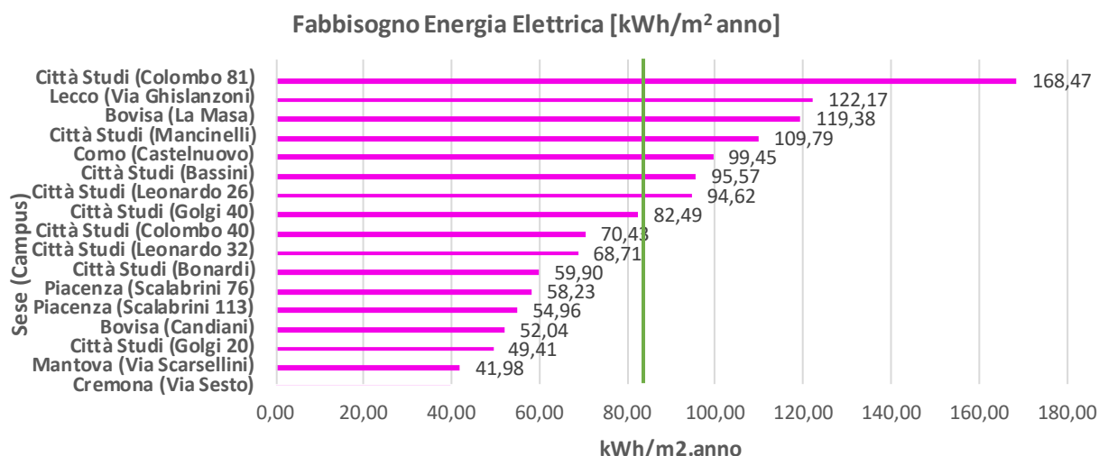
Figura 118. KPI fabbisogno energia elettrica a livello di Campus
