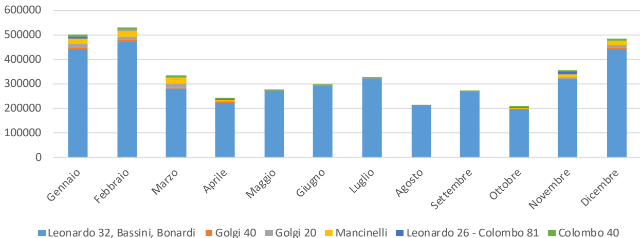
Figura 22. Andamento mensile di consumo di gas naturale [Sm 3 ], Sede di Città Studi
