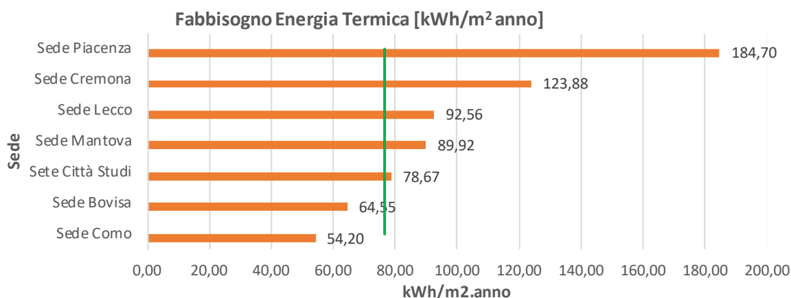
Figura 119. KPI fabbisogno energia termica a livello di Sede
