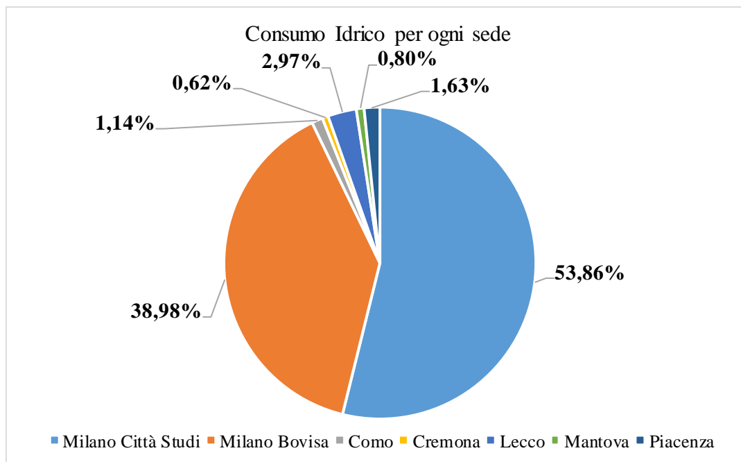
Figura 108 - Consumo idrico percentuale per ogni Sede del Politecnico di Milano
