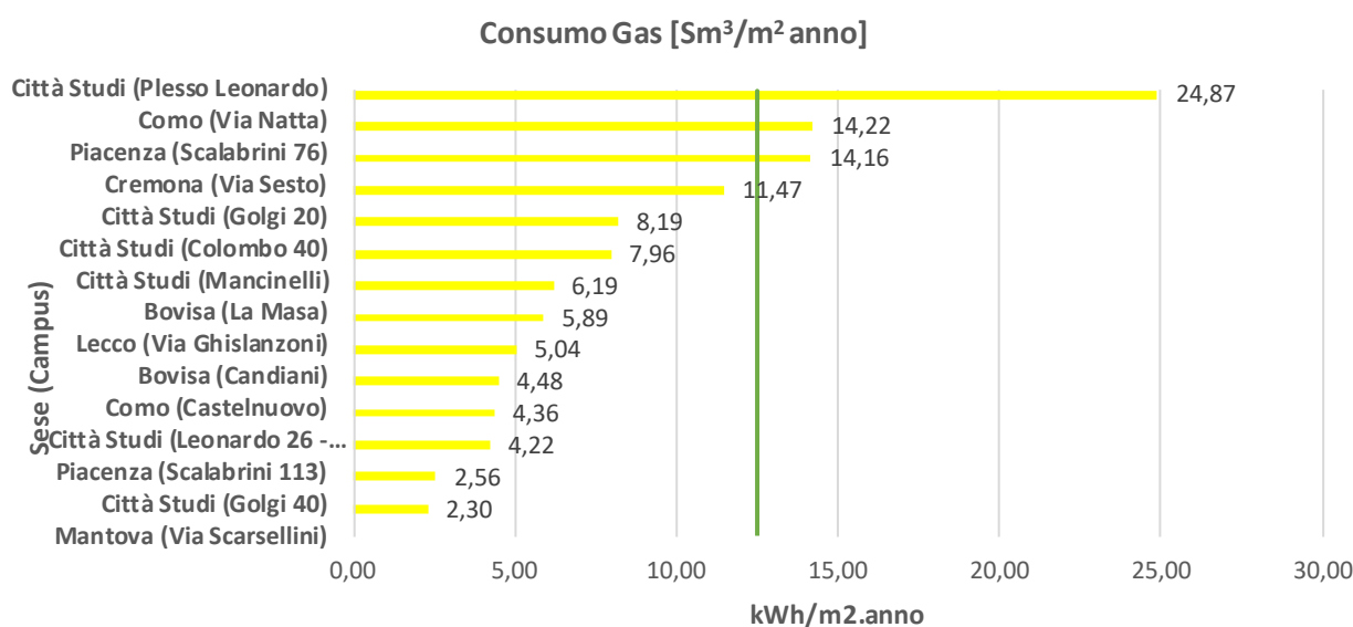
Figura 114. KPI consumo Gas Naturale a livello di Campus
