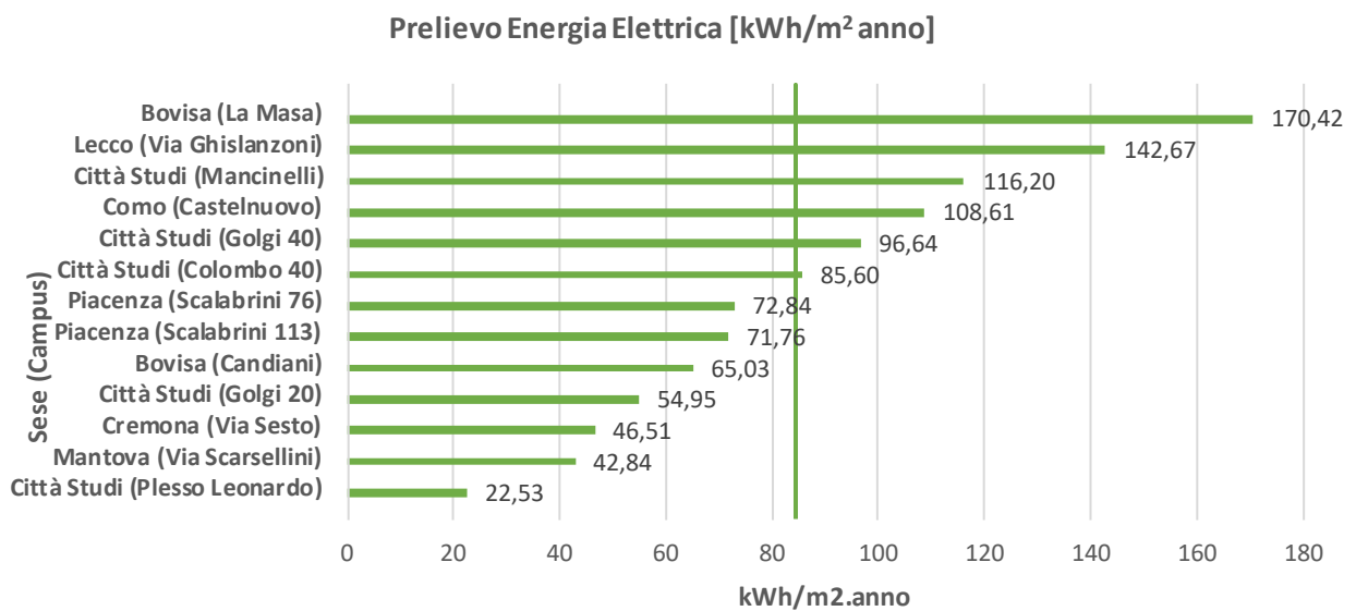
Figura 112. KPI prelievo Energia Elettrica a livello di Campus
