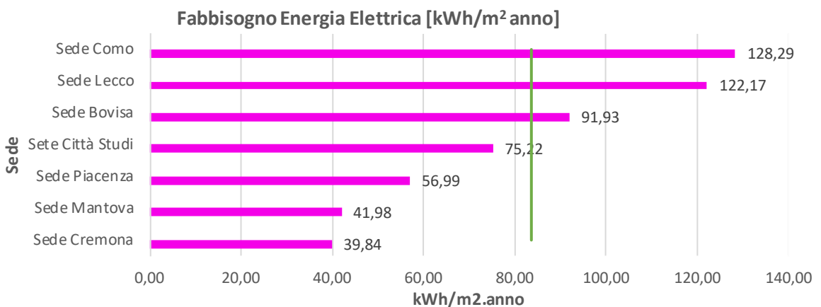
Figura 117. KPI fabbisogno energia elettrica a livello di Sede
