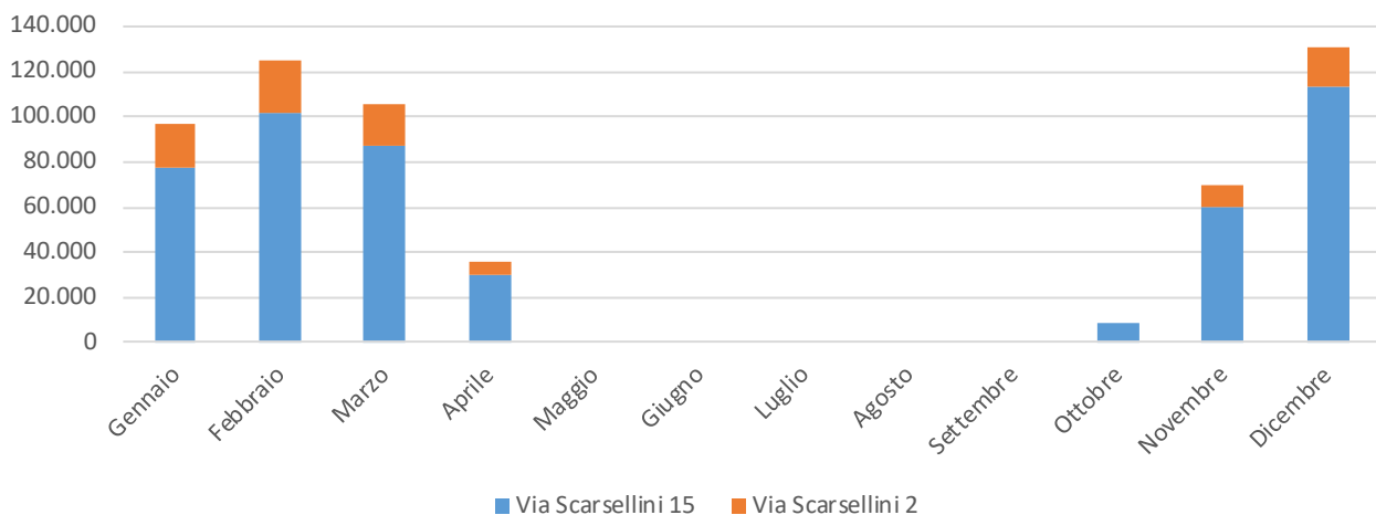
Figura 75. andamento mensile consumo Energia Termica da TLR [kWh], Sede Mantova
