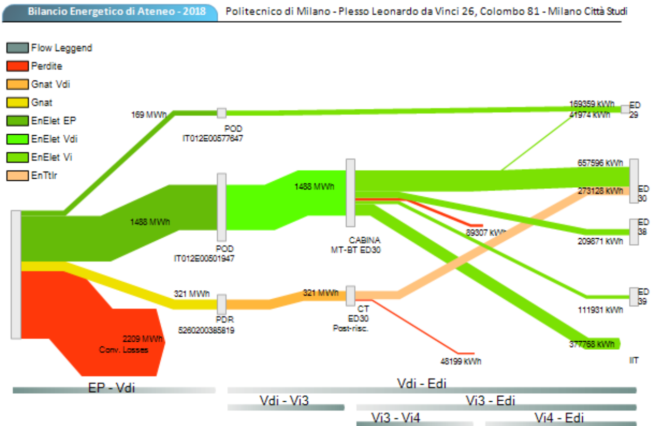
Figura 27. Diagramma di flusso dei vettori energetici, Campus via colombo 81
