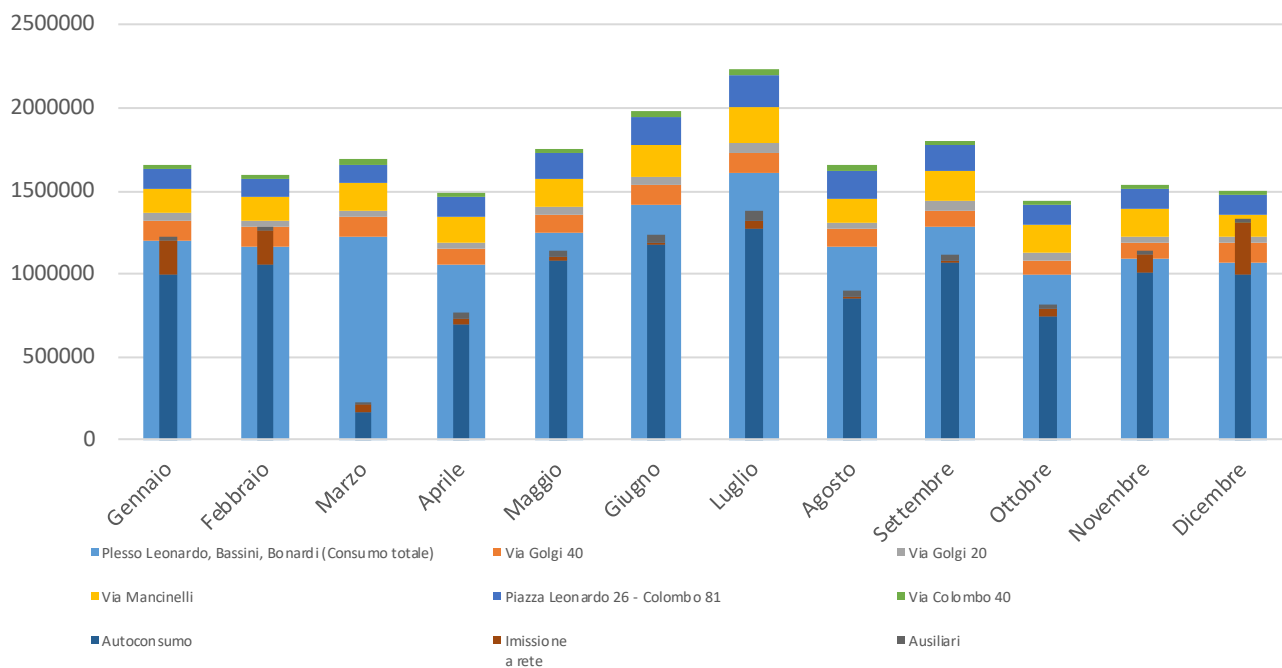
Figura 18. Andamento mensile di consumo e produzione di energia elettrica [kWh], Sede Città Studi
