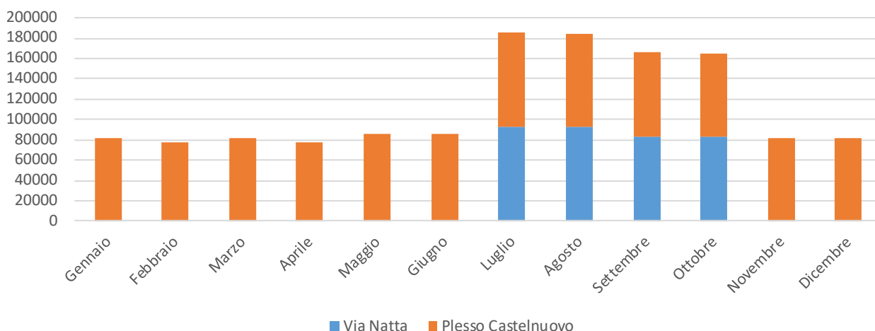
Figura 47. andamento mensile di consumo di energia elettrica [MWh], Sede Como
