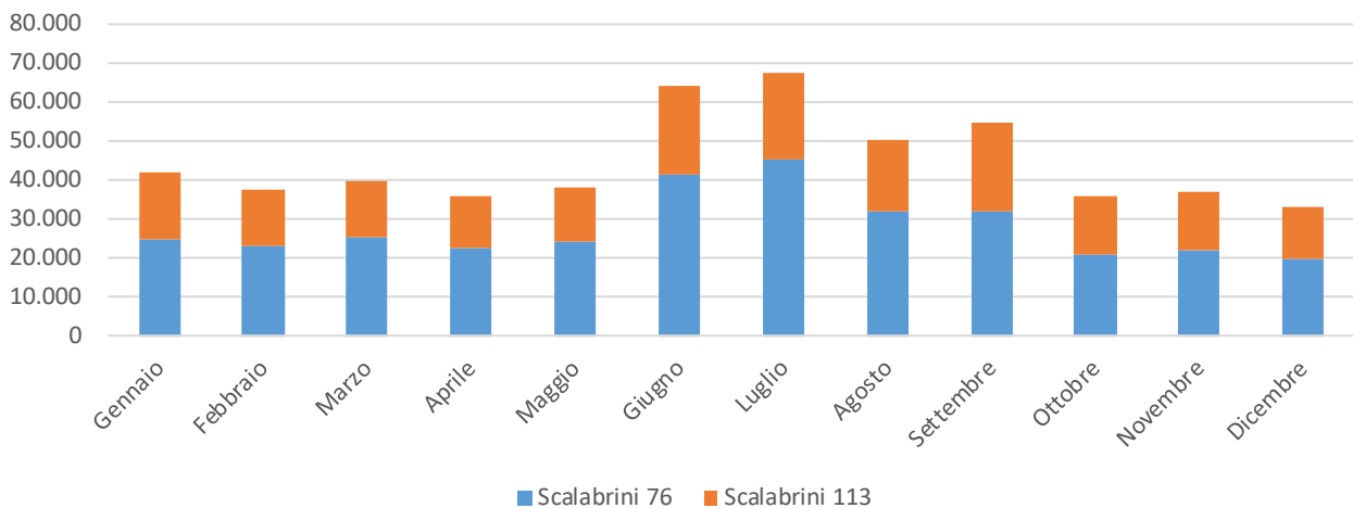
Figura 81. andamento mensile consumo energia elettrica [kWh], Sede Piacenza
