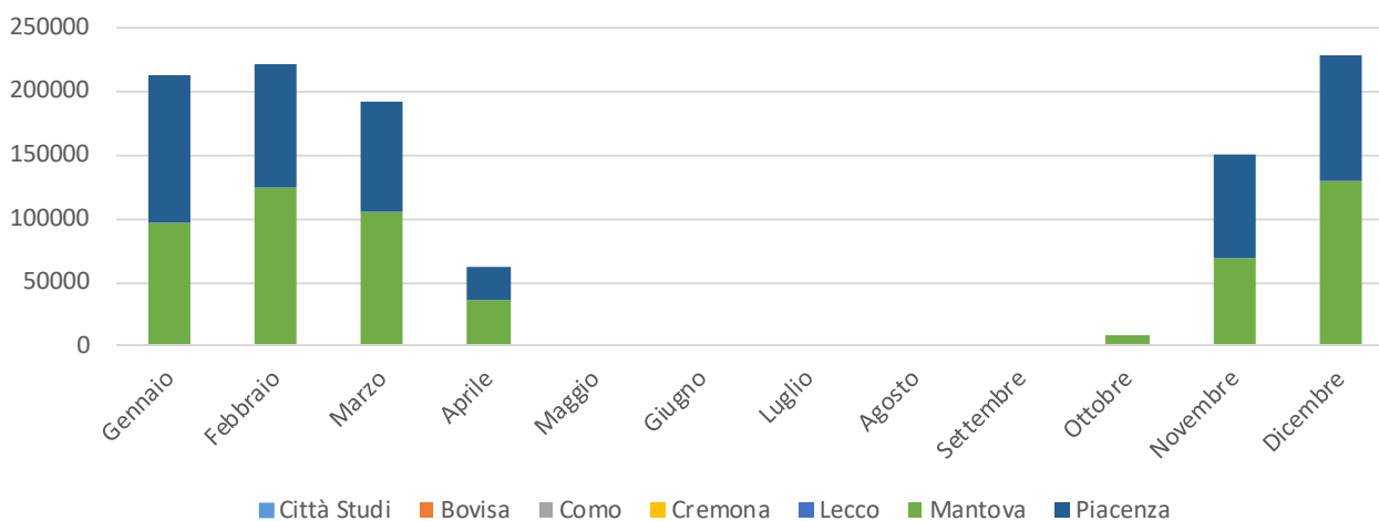
Figura 10. Consumo mensile da TLR esterno [kWh] anno 2018 suddiviso per due Sedi del Politecnico
