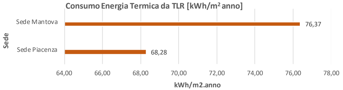
Figura 115. KPI consumo Energia Termica a livello di Sede
