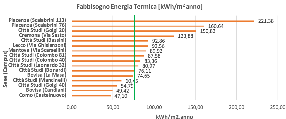
Figura 119. KPI fabbisogno energia termica a livello di Sede
