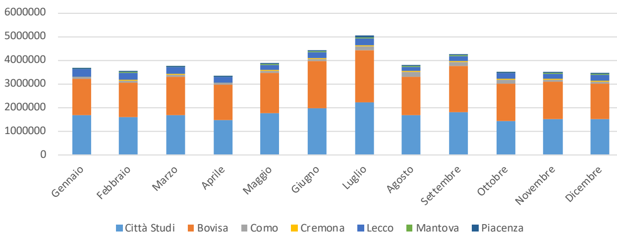
Figura 8 – Consumo mensile Vettore Diretto energia elettrica [kWh] anno 2018, diviso per Sedi
