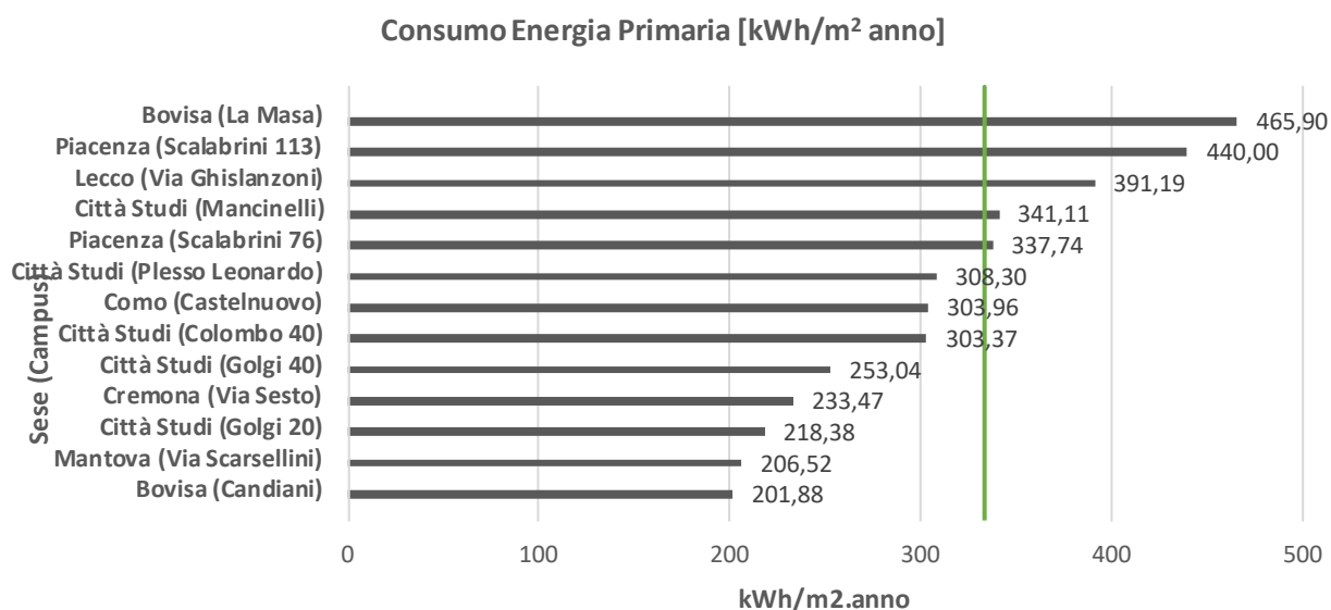
Figura 110. KPI calcolati consumo Energia Primaria a livello di Campus/Plesso
